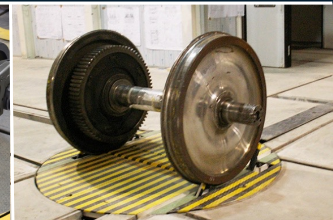
Поворотный круг для колесных пар
